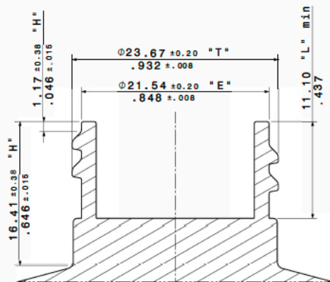
Section cut A-A Scale: 4:1
